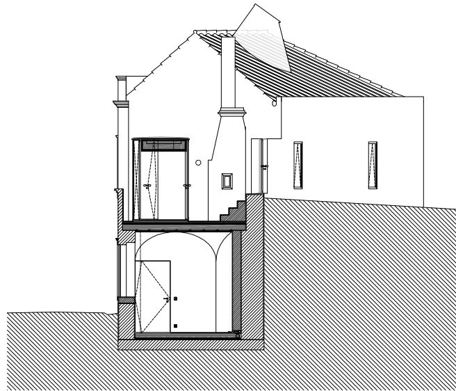
CORTE G G'
