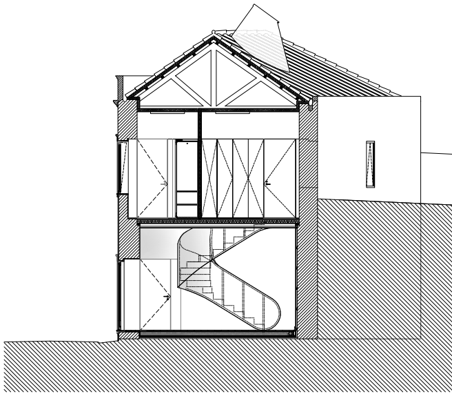
CORTE F F'
