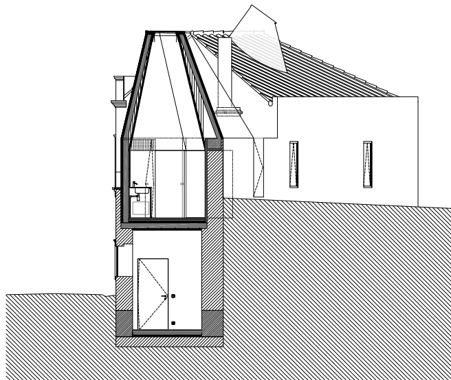
CORTE H H'
