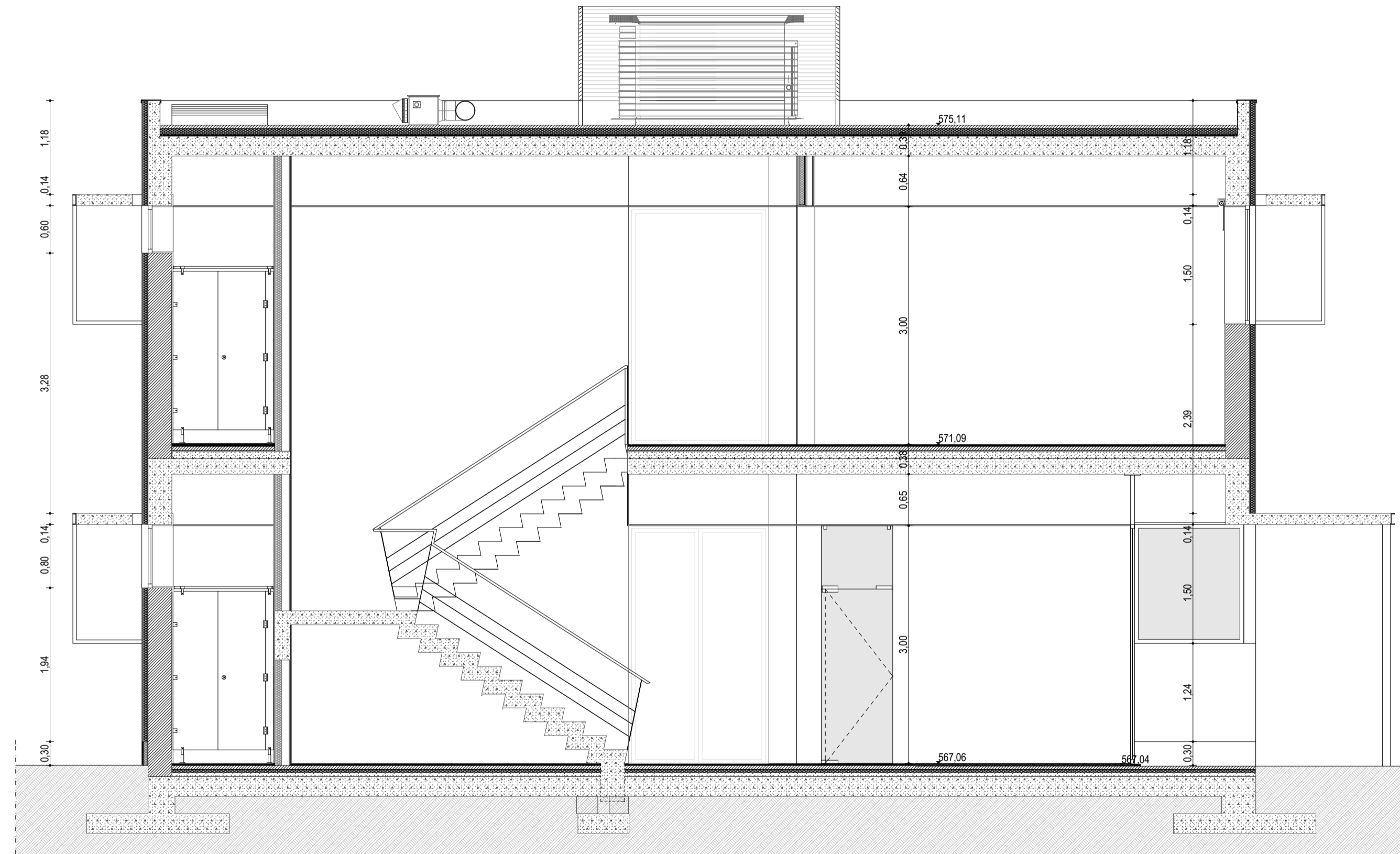
Corte CC'
