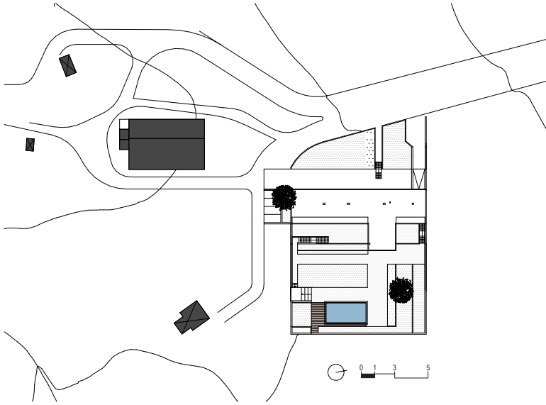
Planta de implantação Site plan
