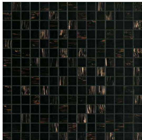
PINATUBO
