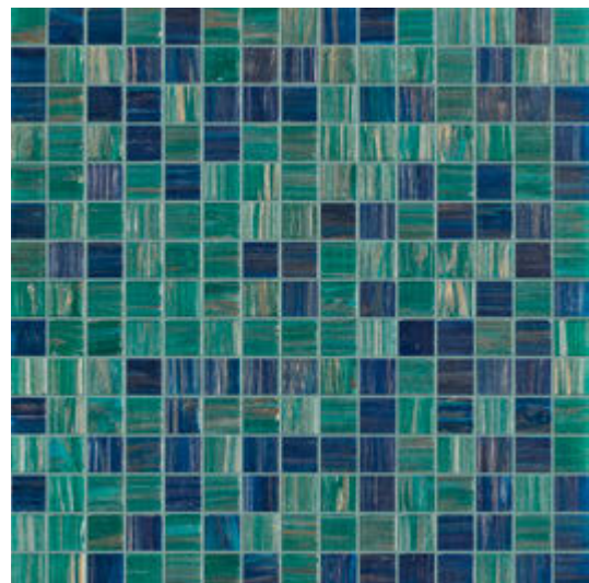
FUJI
