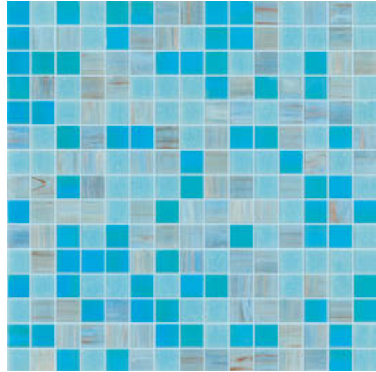
ETNA
