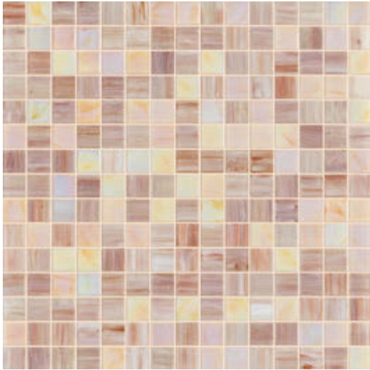
SANTORINI
