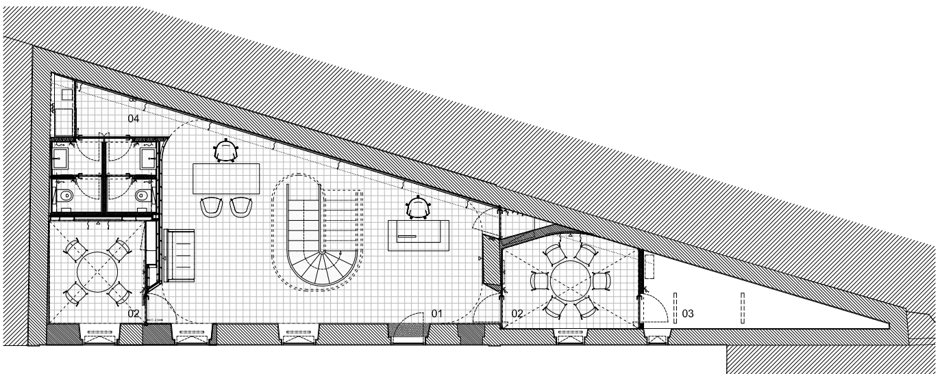
PLANTA PISO 0
