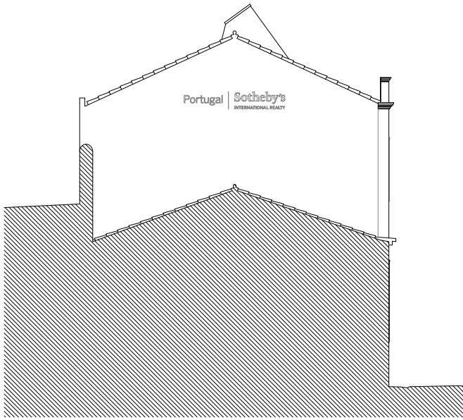
ALÇADO POENTE
