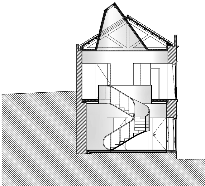
CORTE EE'
