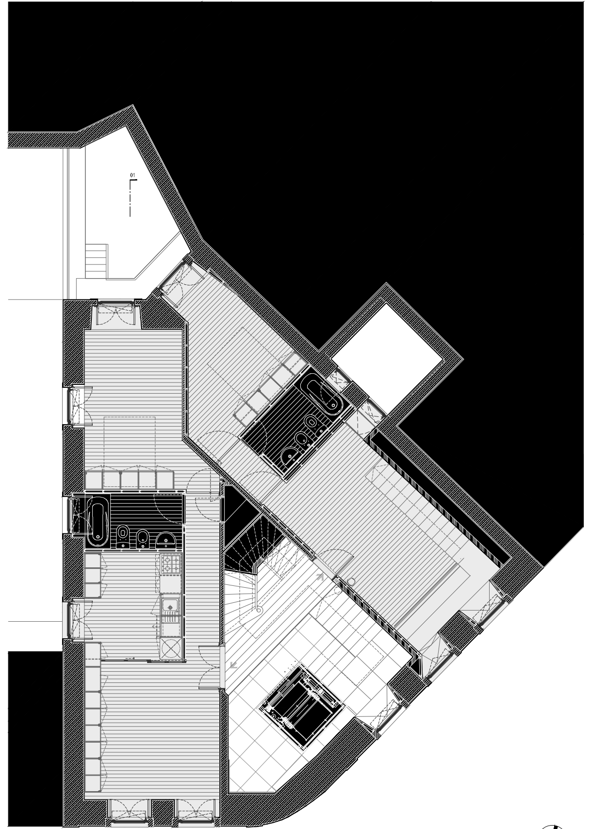
PLANTA PISO 00
