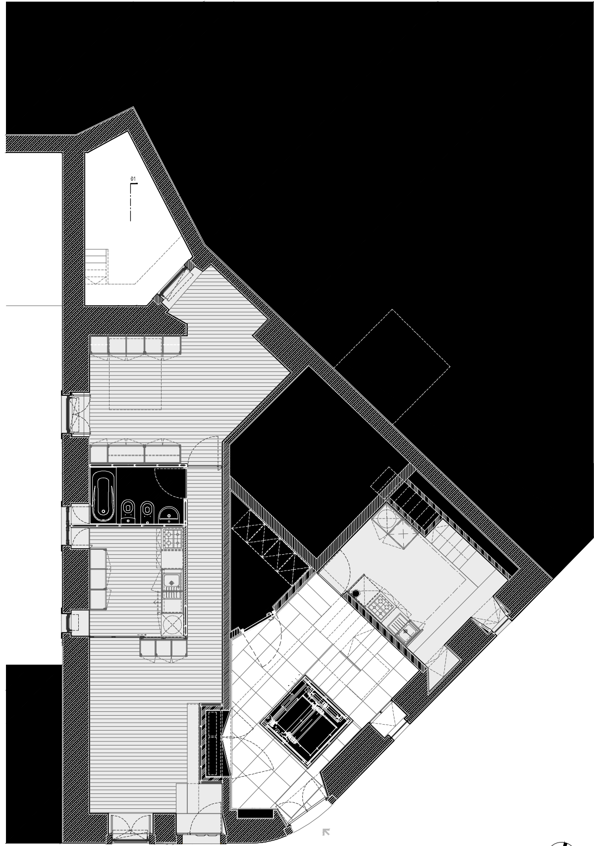
PLANTA PISO -01
