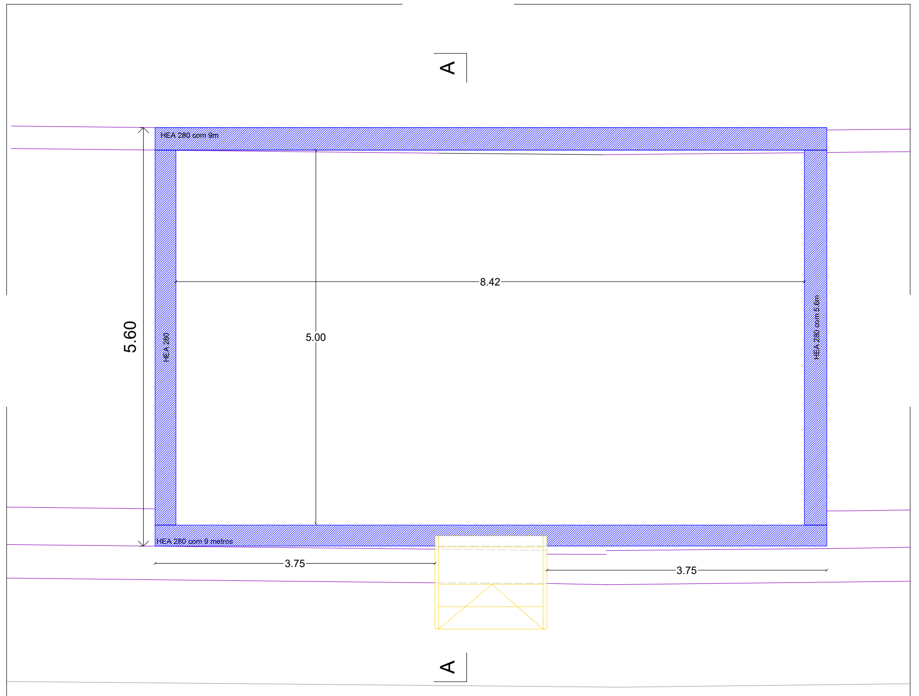
Planta sem rede esc: 1/50
