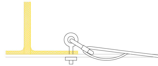
P2 Pormenor da amarração da rede com a viga esc: 1/5
