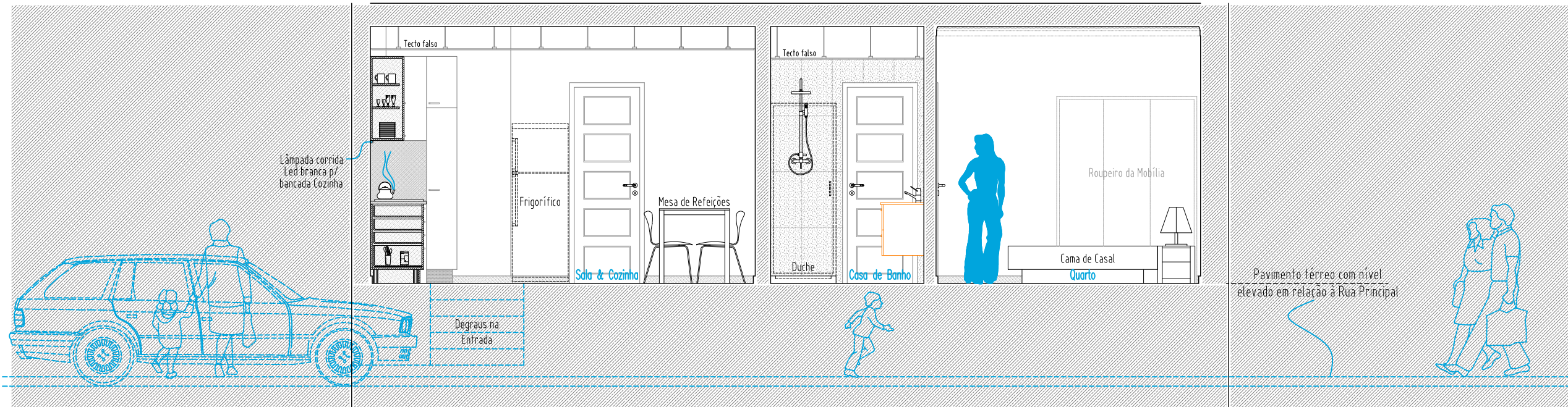
CORTE E-E DA CASA-PÁTEO LISBOETA ESCALA: 1/50
