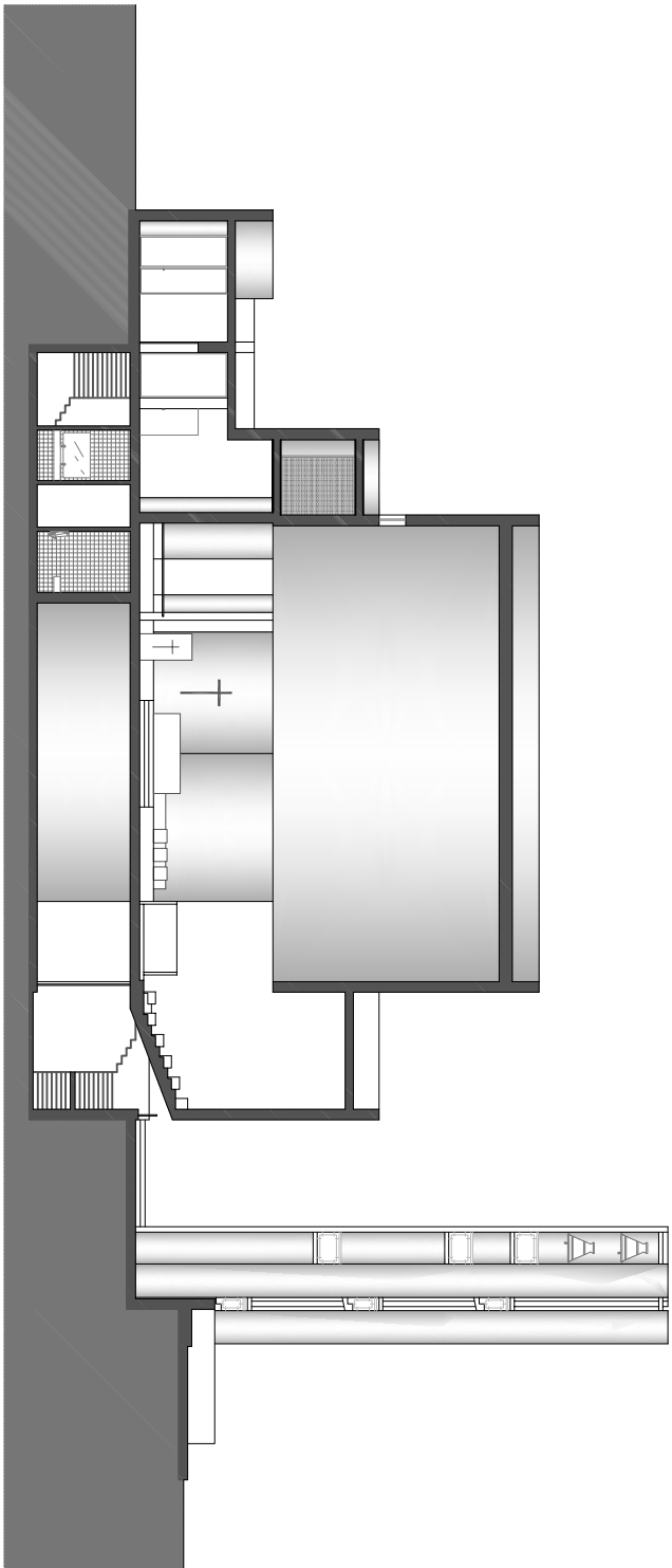
0m 1m 2m Corte B
