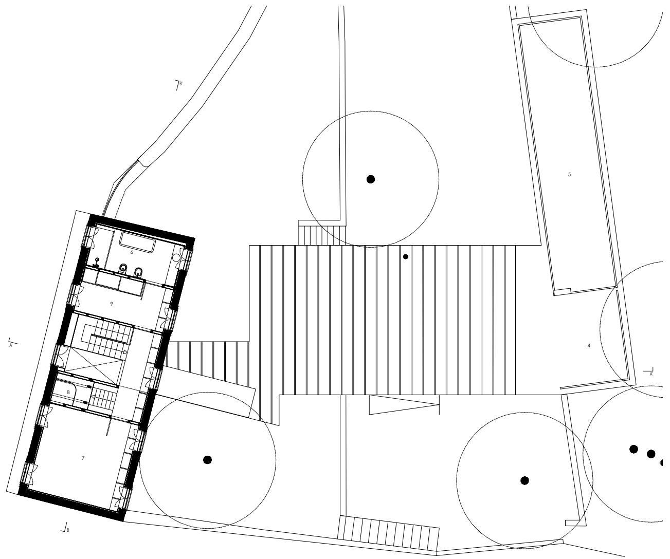
planta piso 2
