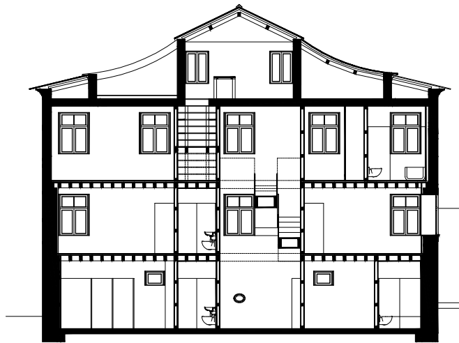
corte B
