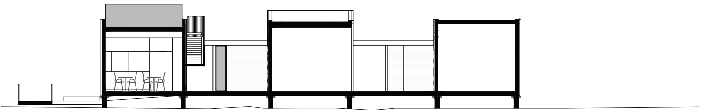
CORTE BB'
