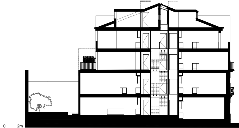
0 2m Corte A Section A
