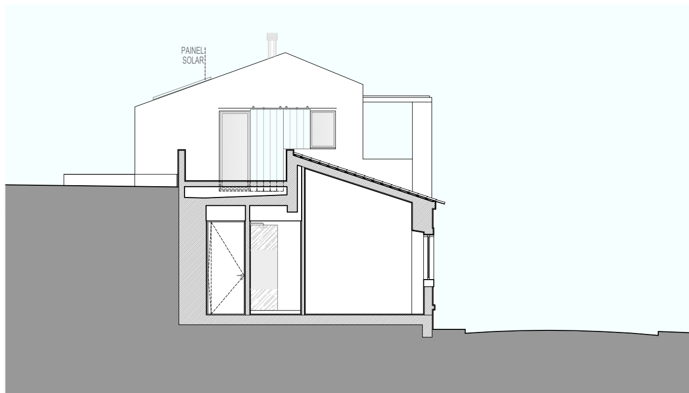
corte 2.2 . 1.100
