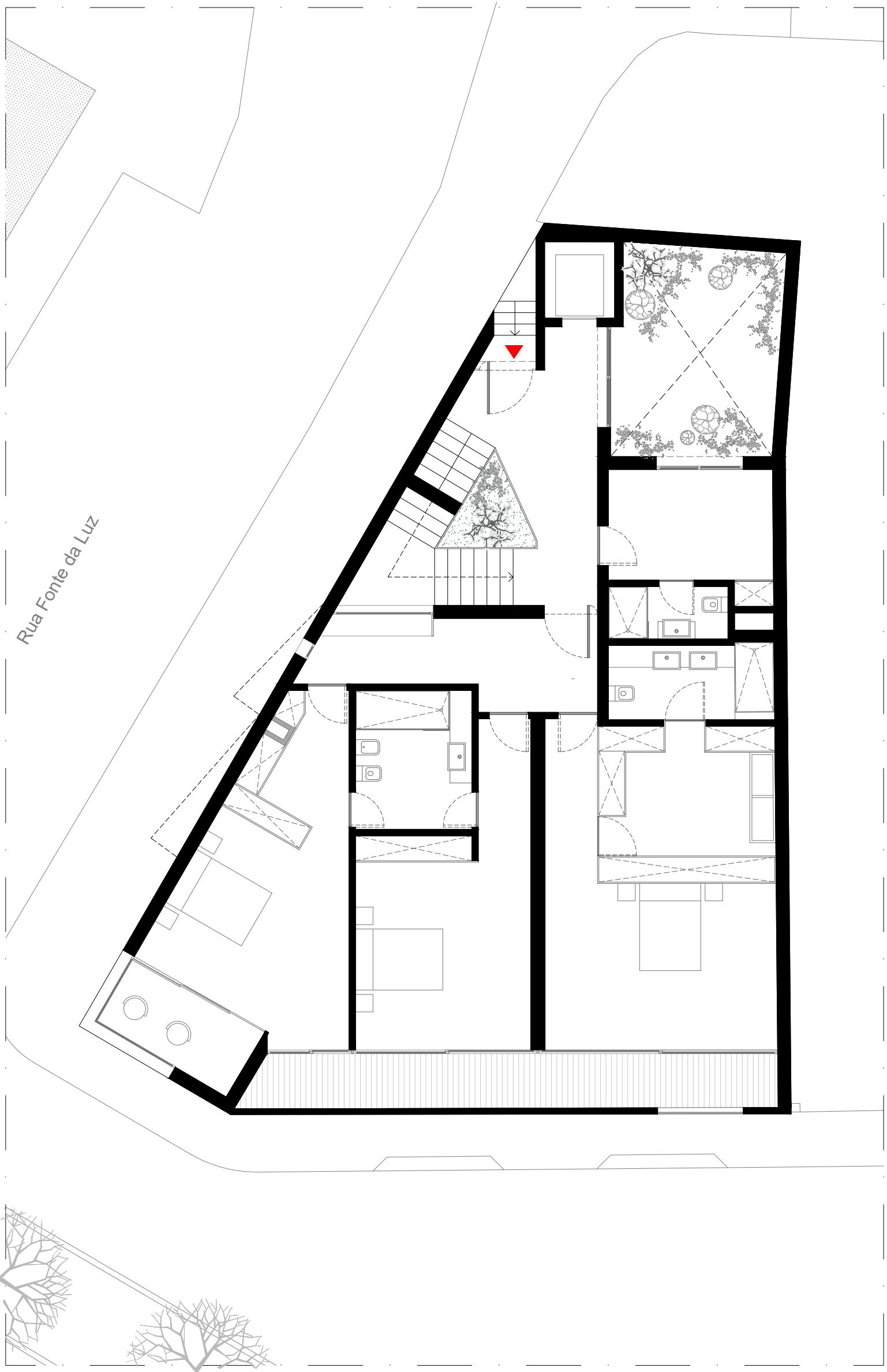
PLANTA PISO 1
