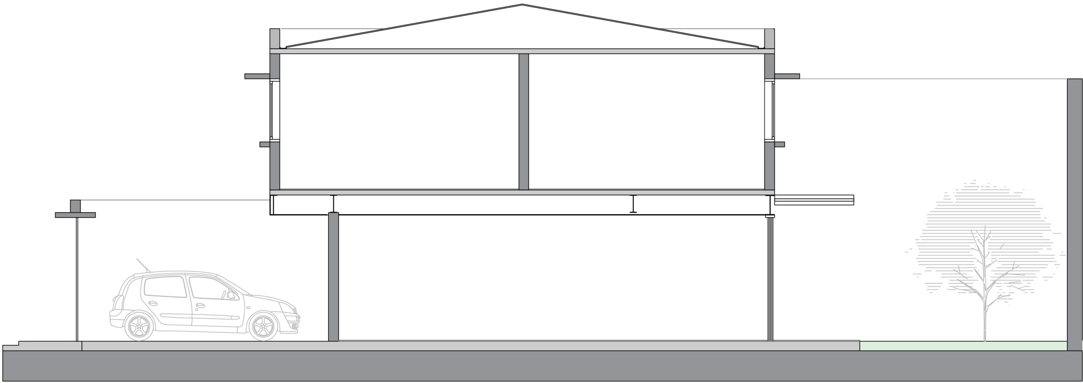
CORTE 01 ESCALA:1:50
