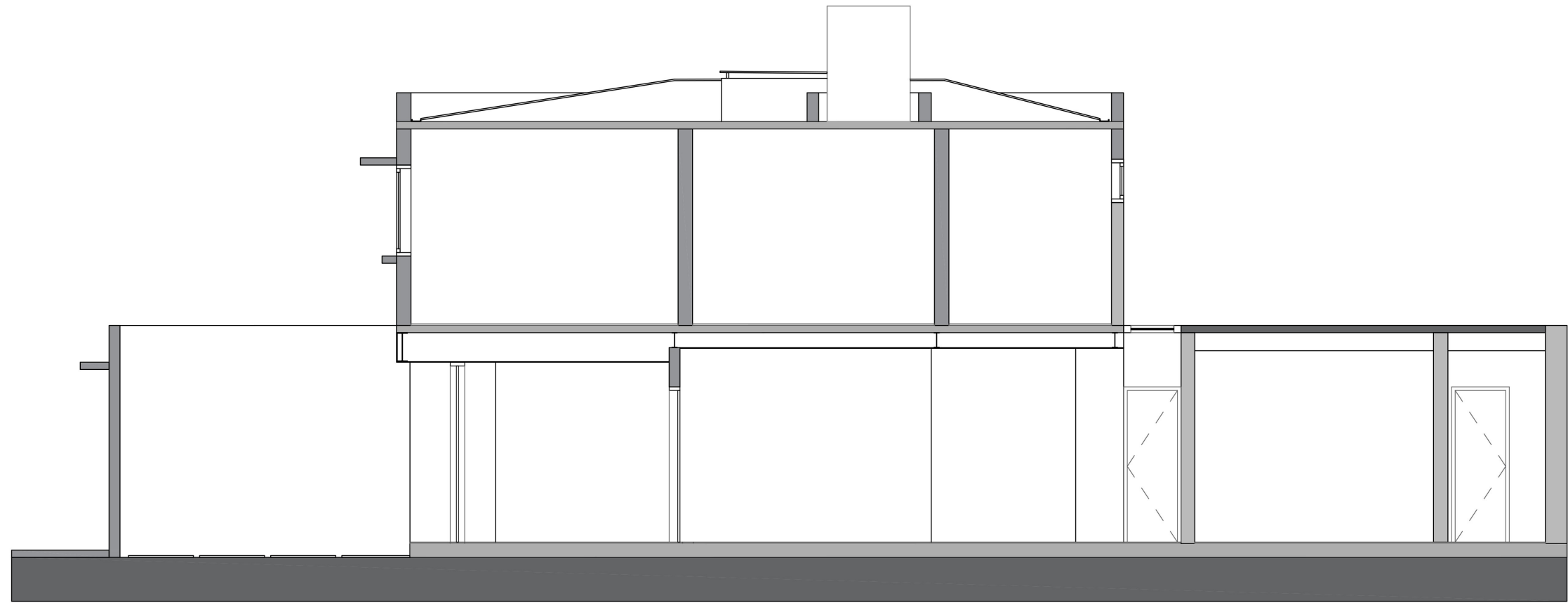
CORTE 02 ESCALA:1:50
