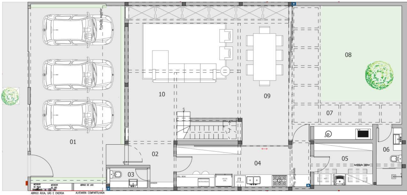
PLANTA TÉRREO
