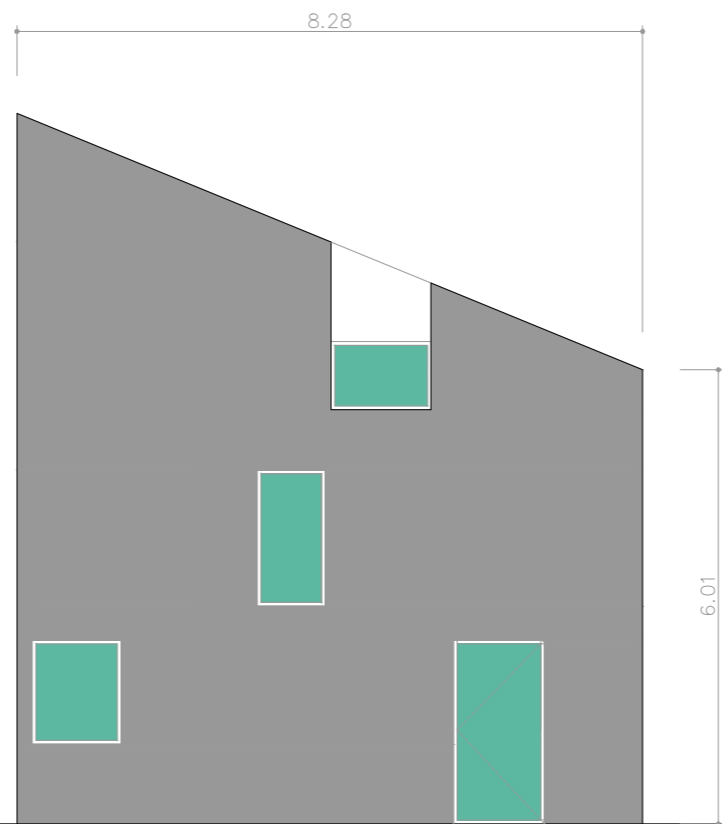
Alçado Poente
