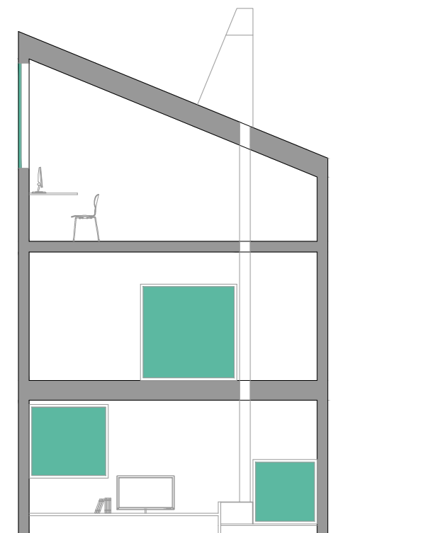
Corte E-F
