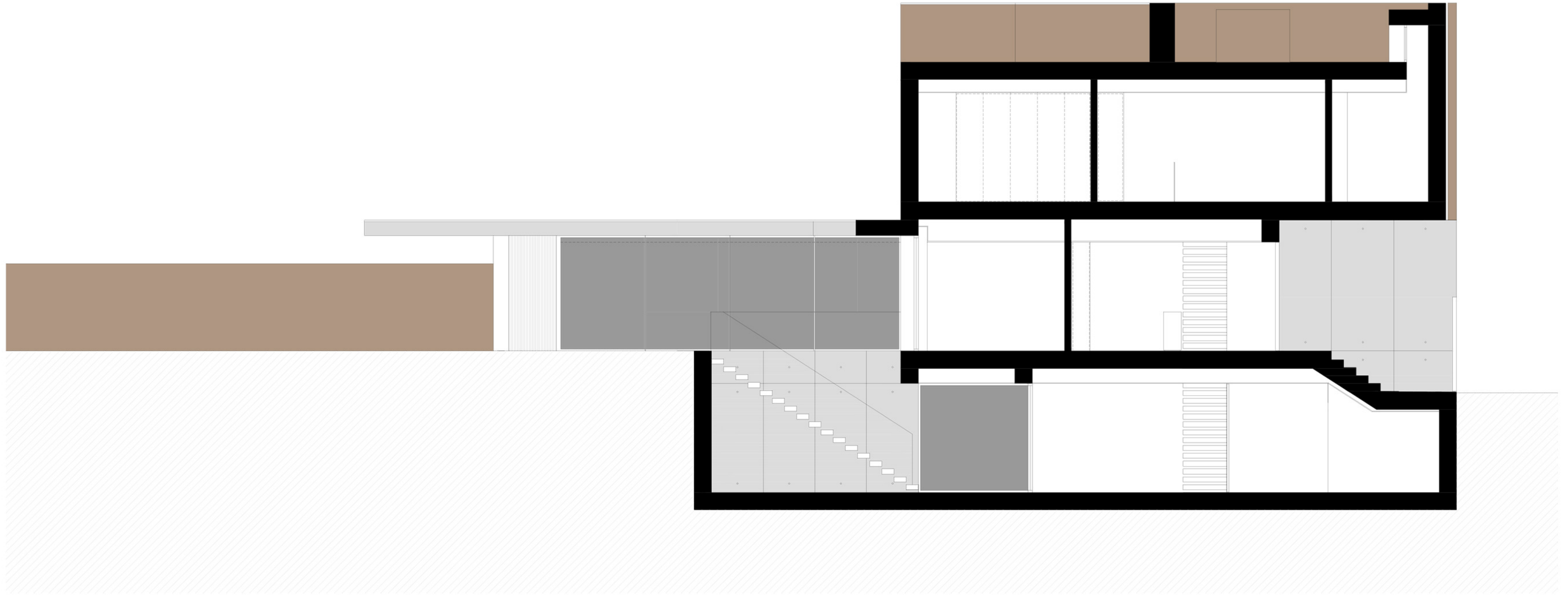
0 1 5m longitudinal section
