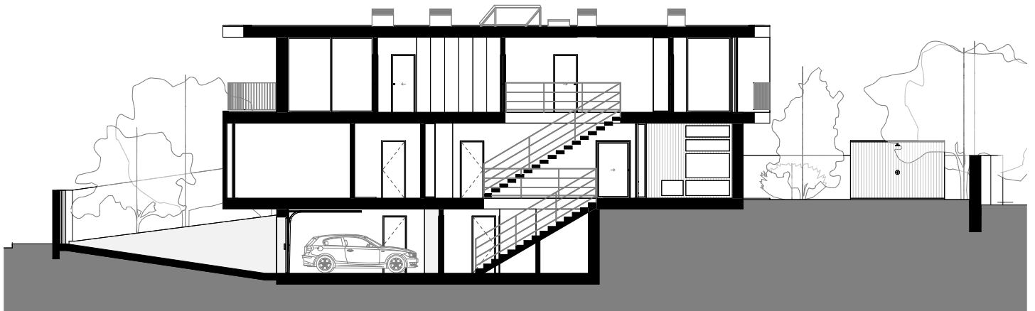
CORTE 01
