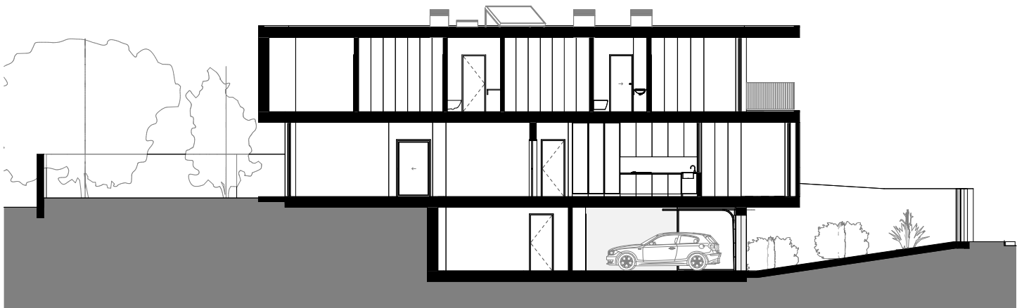
CORTE 02
