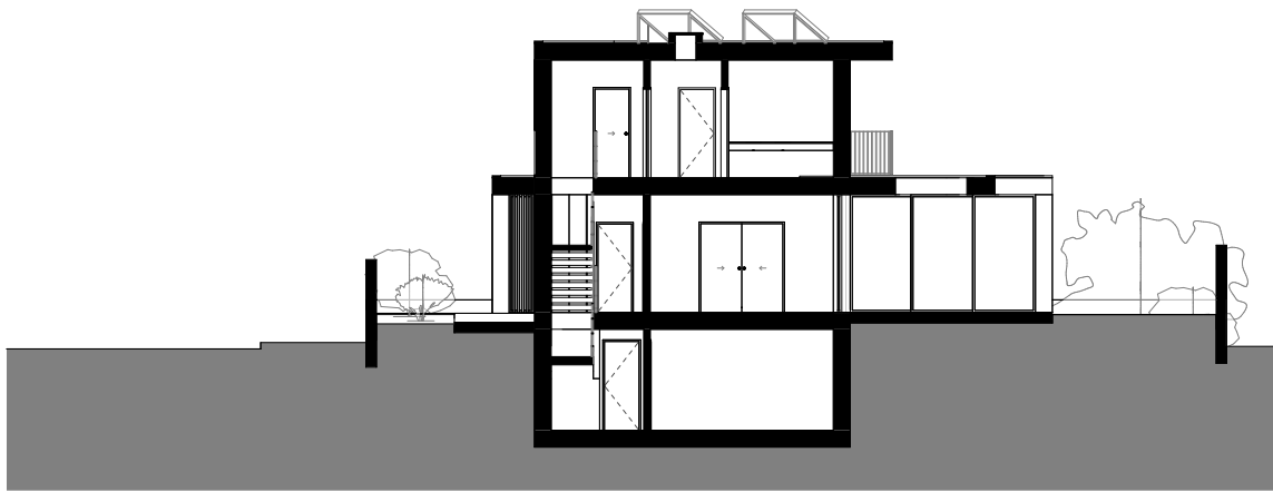
CORTE 05
