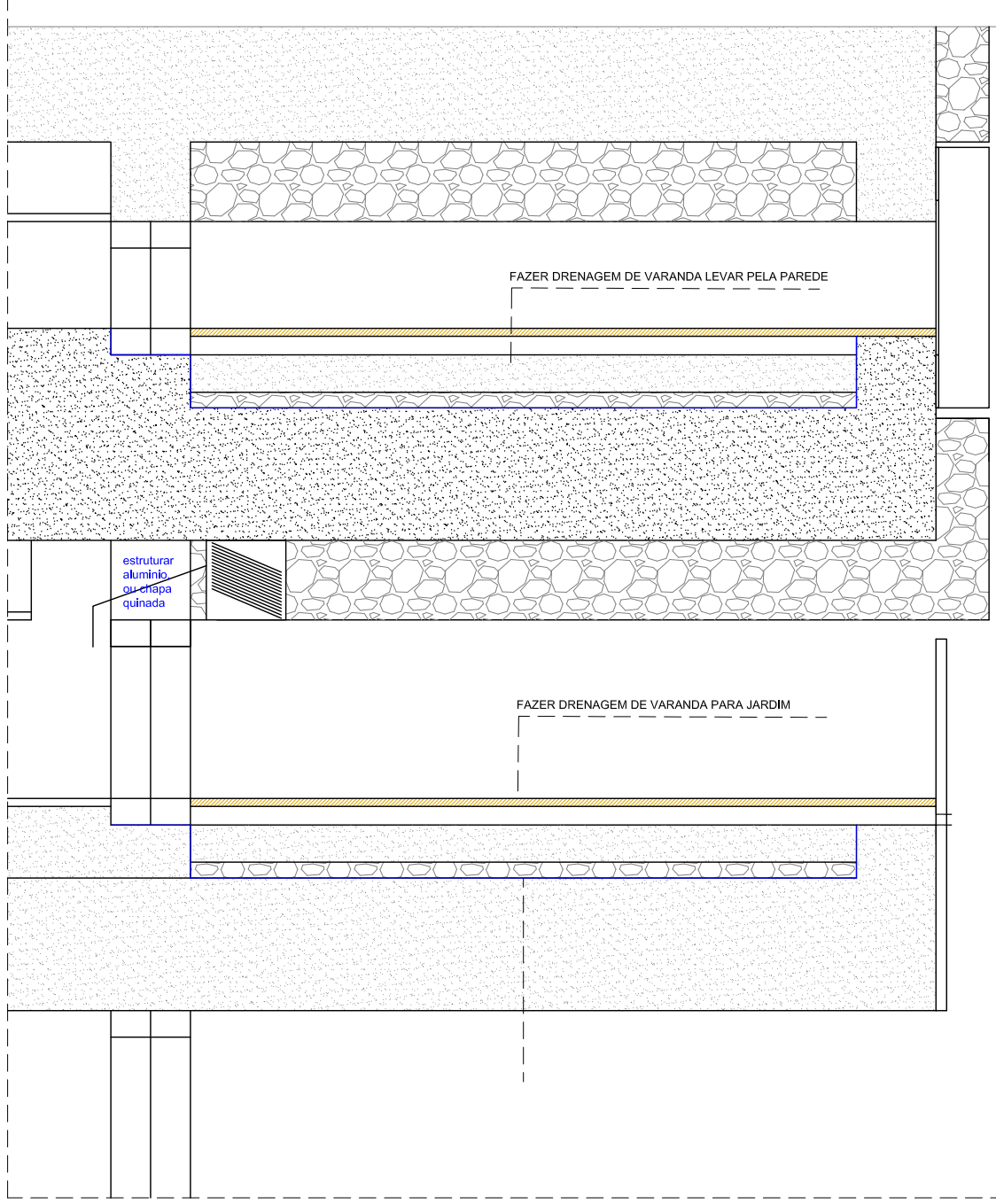
PORMENOR ALÇADO POENTE
