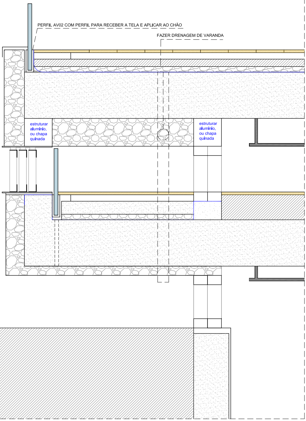
PORMENOR RÓMULO NETO ( CAVE/ VARANDA QUARTO/ VARANDA SALA)
