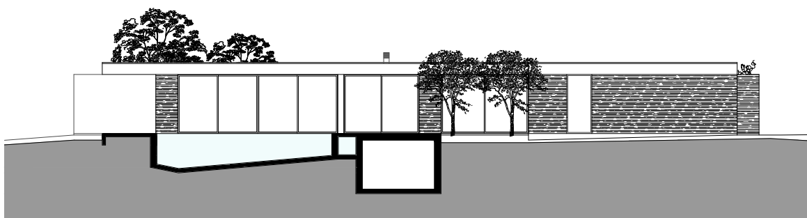
ALÇADO SUL
