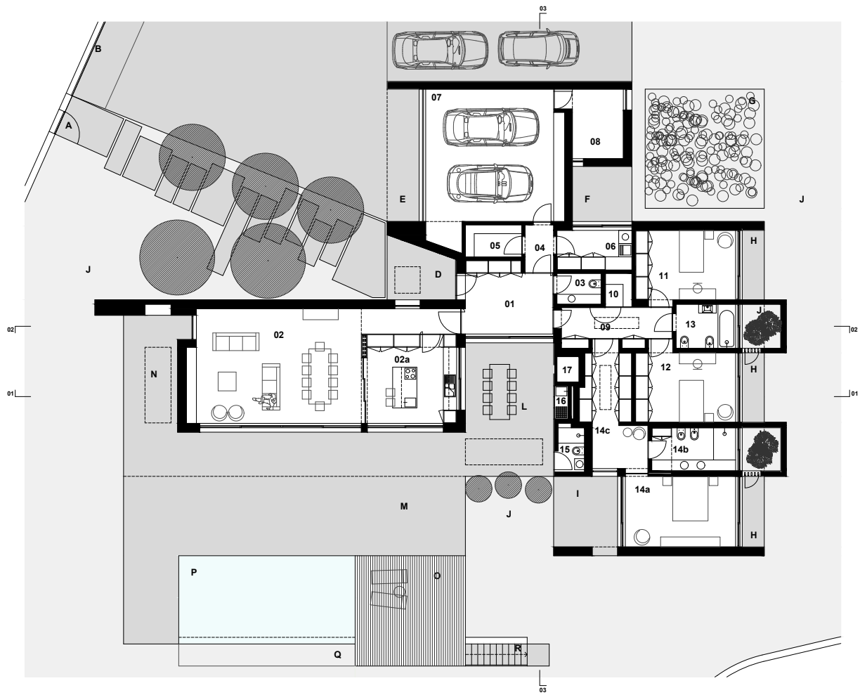
PLANTA DO RÉS-DO-CHÃO
