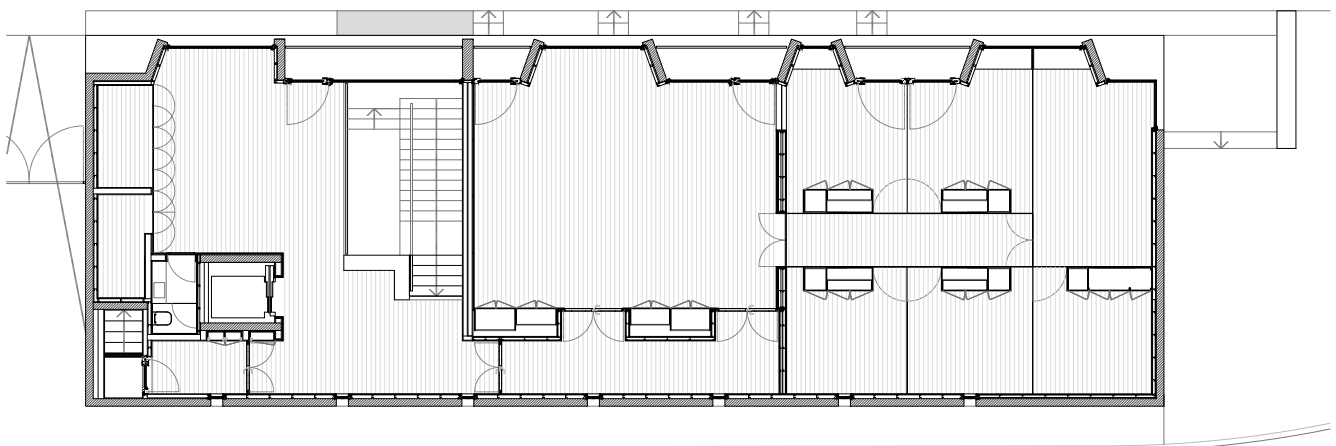
planta piso 1
