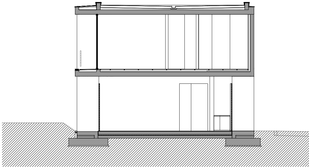
corte b
