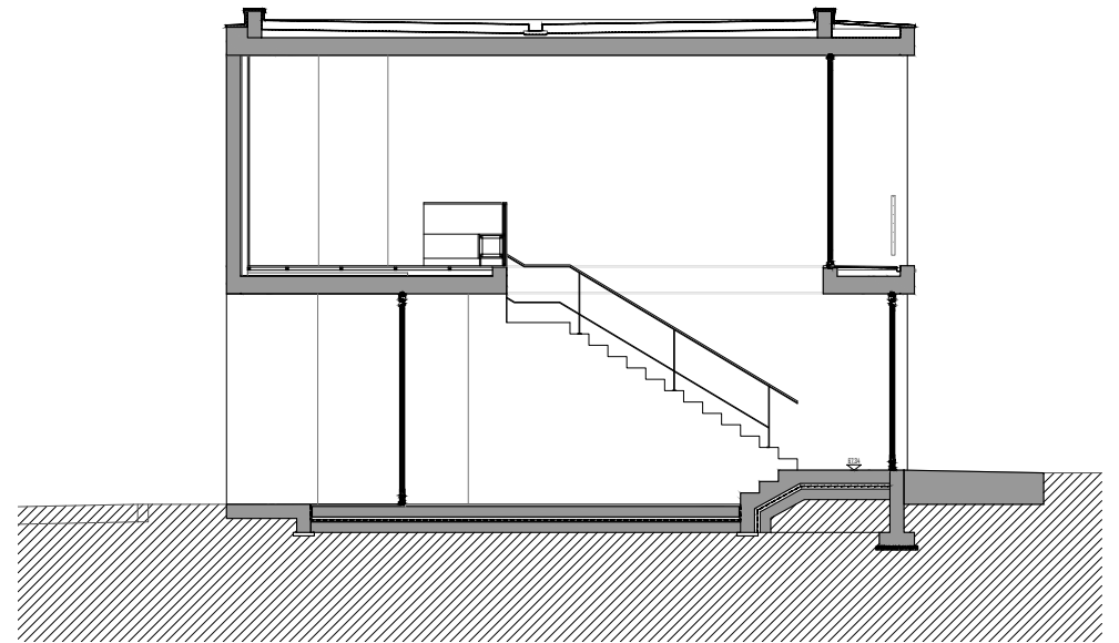
corte c
