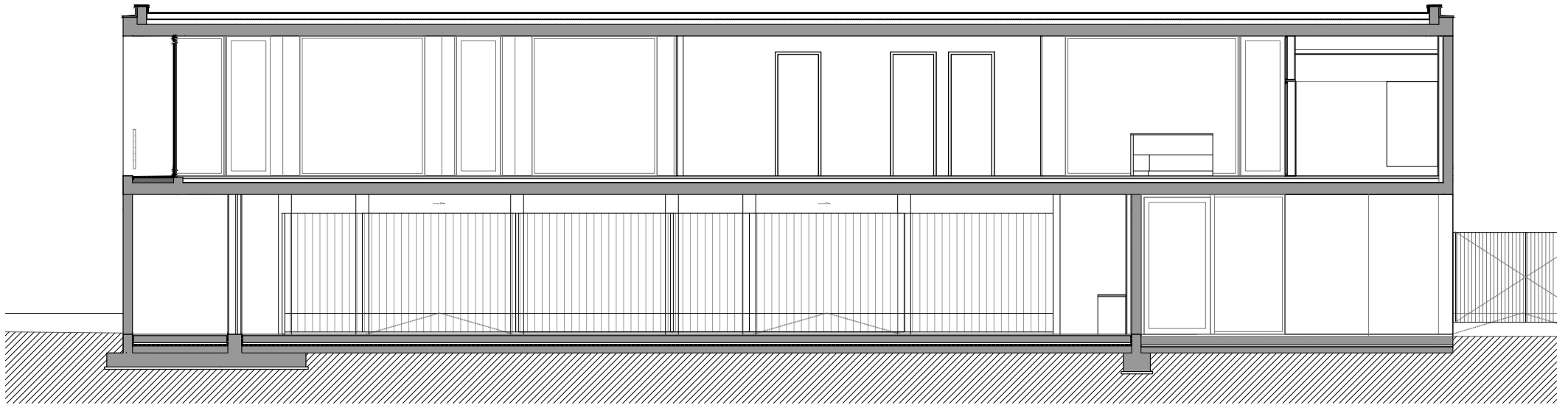
corte a
