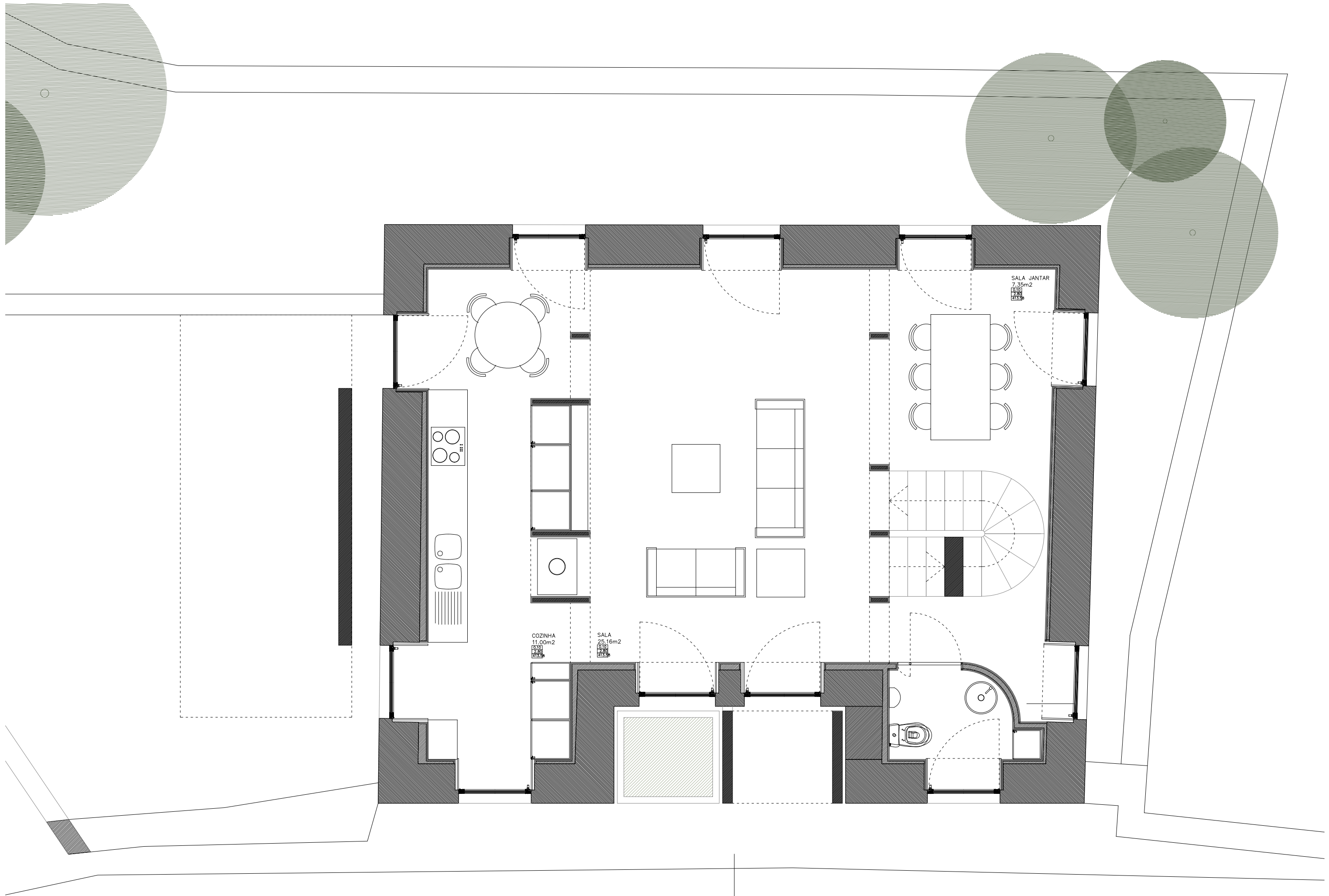
Planta Piso 0
